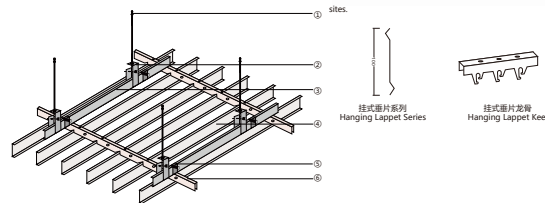
安装示意图
