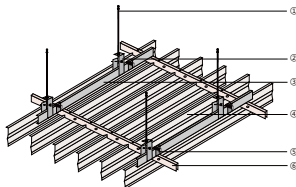
安装示意图
