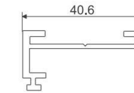
HLB-075 顶层板收口
