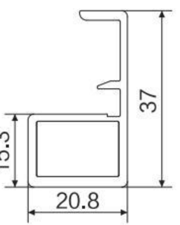
壁厚: 2.3mm 米重: 0.5kg/m
