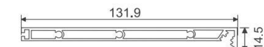
HLB-076 顶层底板
