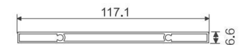
HLB-077 隔板
