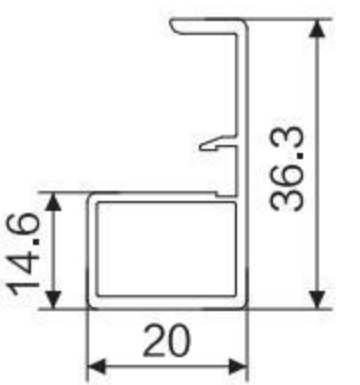
HLB-003 F拉手B款
