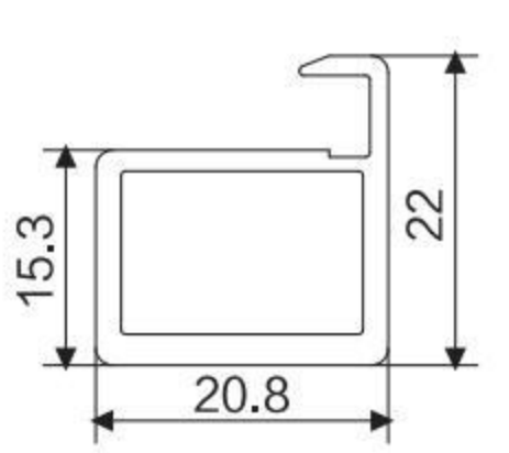
壁厚: 2.3mm 米重: 0.39kg/m
