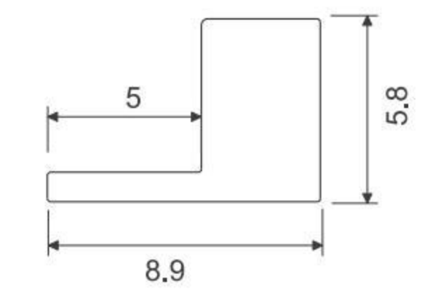
HLB-080 转5转换条
