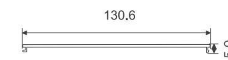
HLB-078 侧板盖板
