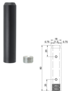
B款套座 11管用 Type B Socket Base - For 11 mm Tube
