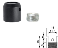
D款套座 11管用 Type D Socket Base - For 11 mm Tube
